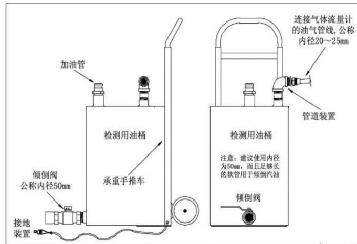
图 C.2 检测用油桶部件安装示意图
