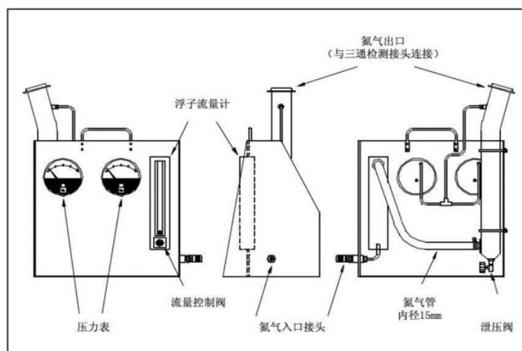
图 A.1 液阻和密闭性检测装置示意图
