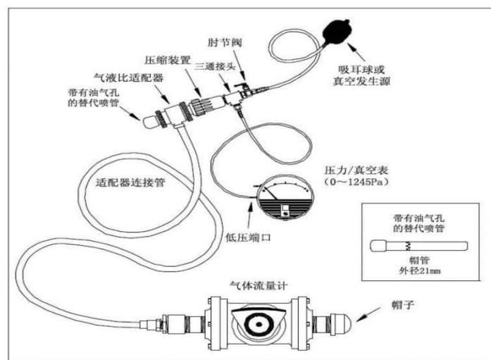
图 C.4 气液比适配器泄漏检测装置安装示意图
