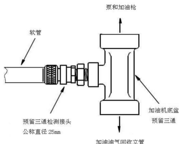
图 A.2 三通检测接头示意图
