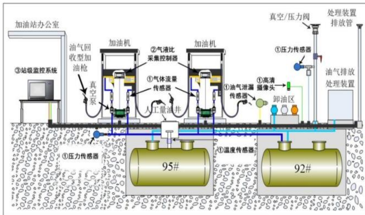
图 E.1 在线监控系统
